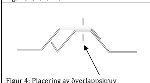
Figur 4: Placering av överlappskruv
